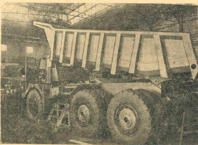
Attēlā: pirmā pašizkrāvēja MAZ-530 montēšana.
